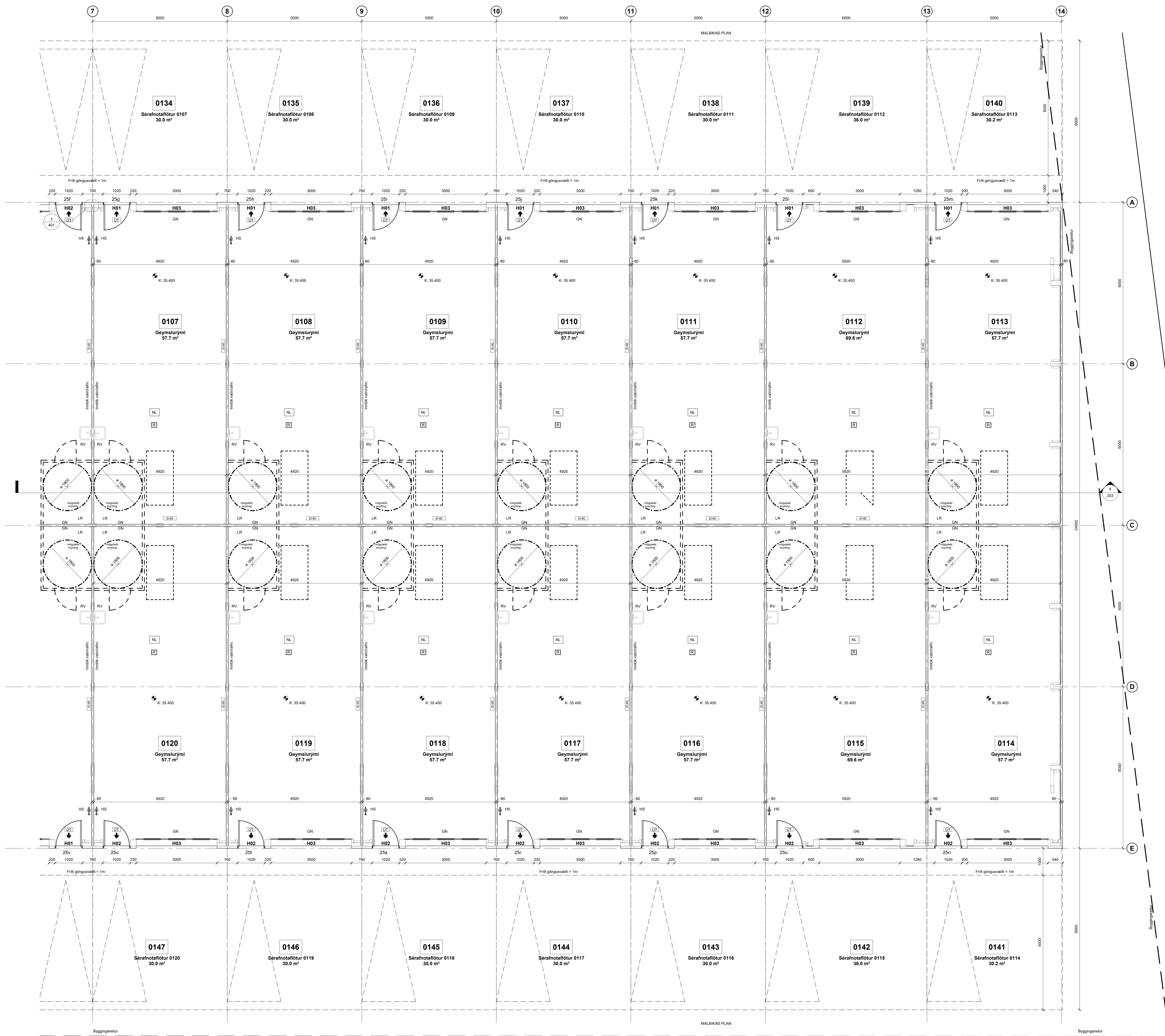
GRUNNMYND 1.HÆÐ - Hluti 7-14 1 : 50
